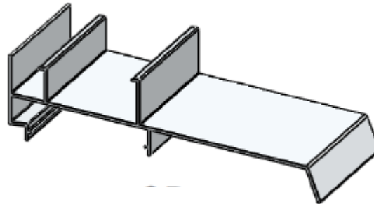
Sillar con alfajía - EXA581
